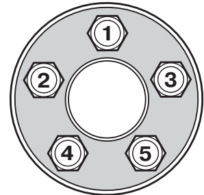
5 - Lug Pattern
